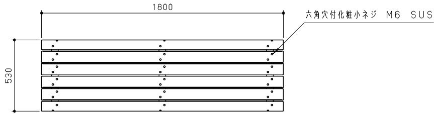
平面図 S = 1/20
