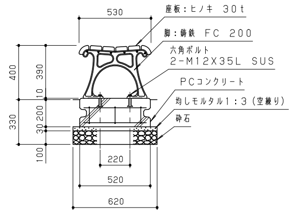
側面図 S = 1/20
